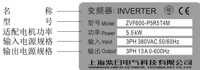
图 2-2 变频器铭牌
