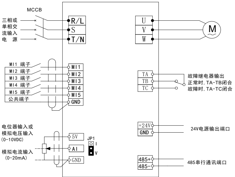
图 3-1 基本配线图
