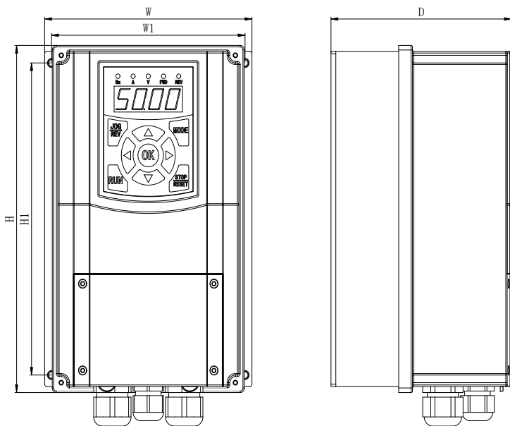
图 7-2 变频器尺寸示意图
