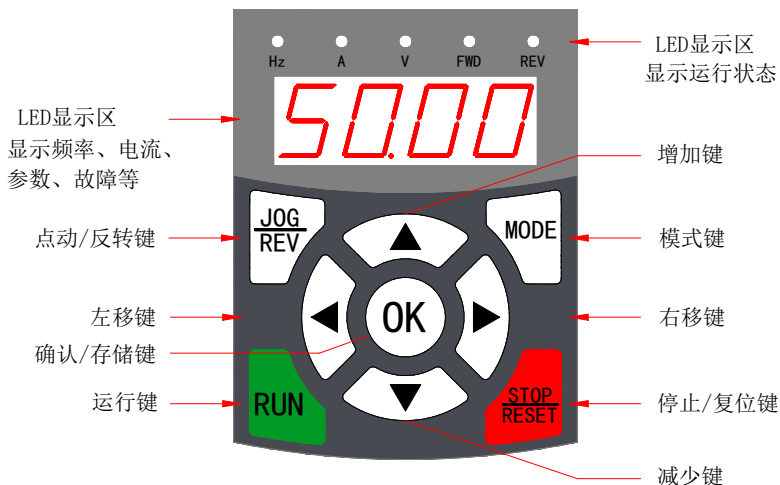
图 4-1 E-600G 面板示意图
