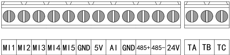
图 3-3 控制电路端子
