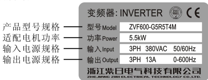
图 2-2 变频器铭牌
