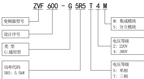
图 2-1 变频器型号说明
